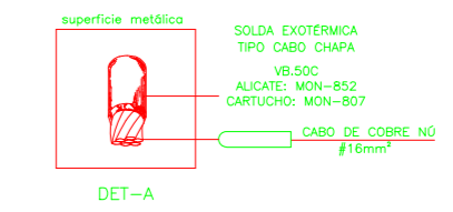
DETALHE - 04 INTERLIGANDO USADO COMO DESCIDA NATURAL COBRE #35mm2 AO ATERRAMENTO SEM ESCALA
