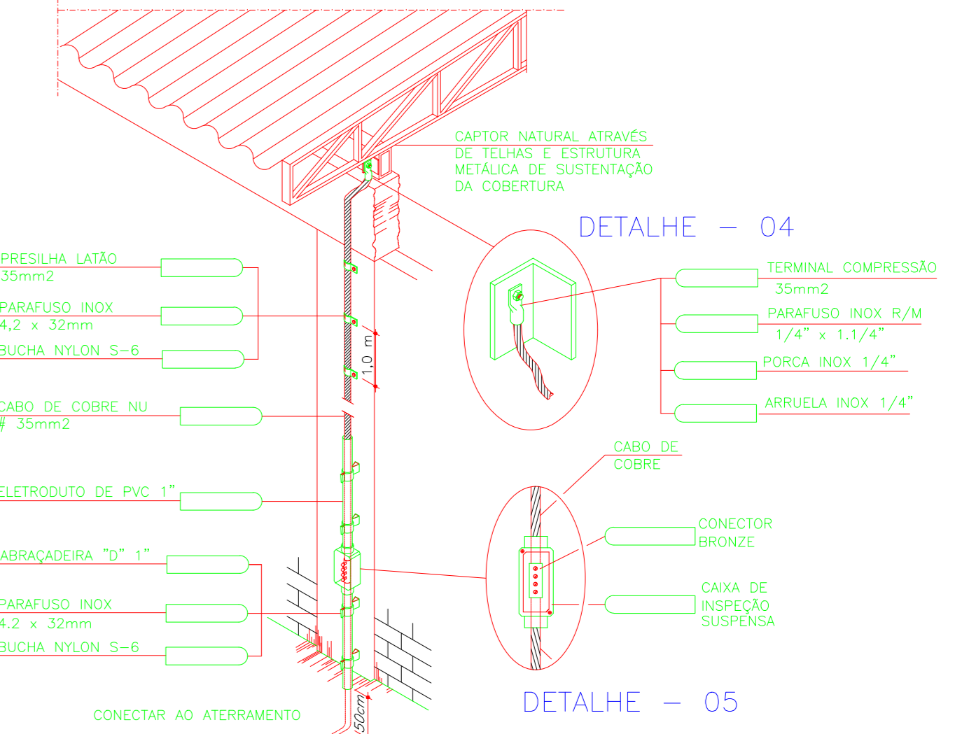
DETALHE - 04 DESCIDA APARENTE COM CABO DE COBRE NÚ #35mm2 TELHADO METÁLICO AO ATERRAMENTO SEM ESCALA
