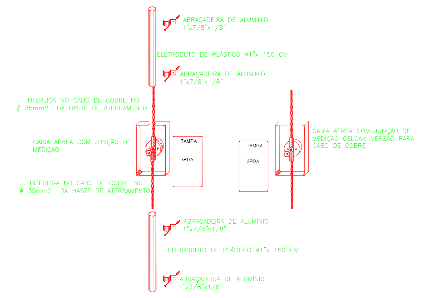
DETALHE - 05 DETALHE DA JUNTA MÓVEL SEM ESCALA
